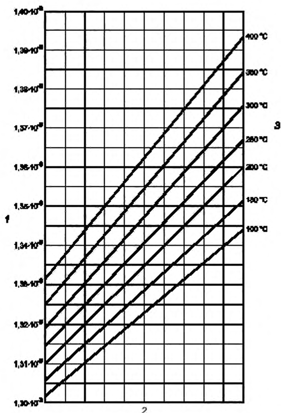
1 — средняя удельная теплоемкость продуктов сгорания, МДж/(м 3 · К); 2 — концентрация CO 2 в продуктах сгорания, %; 3 — температура продуктов сгорания, °C
