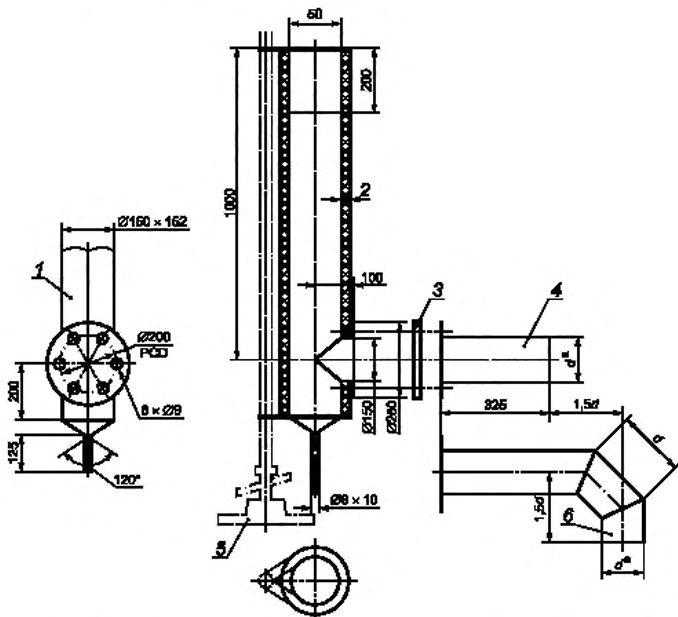
1 — труба дымохода из нержавеющей стали, 2 — теплоизоляция (стекловолокно плотностью 64 кг/м³); 3 — прокладка; 4 — соединительная труба из нержавеющей стали; 5 — опорная стойка; 6 — соединительная труба из нержавеющей стали
