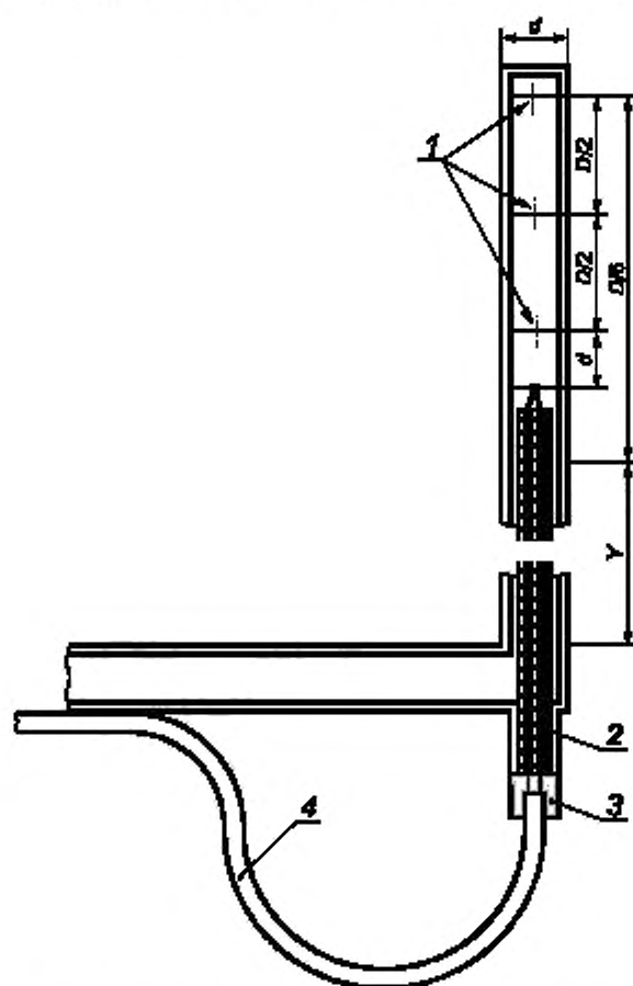
1 — точки отбора проб; 2 — керамическая трубка с двумя каналами; 3 — изолирующий цемент, 4 — провода термопары (хромель — алумель)
