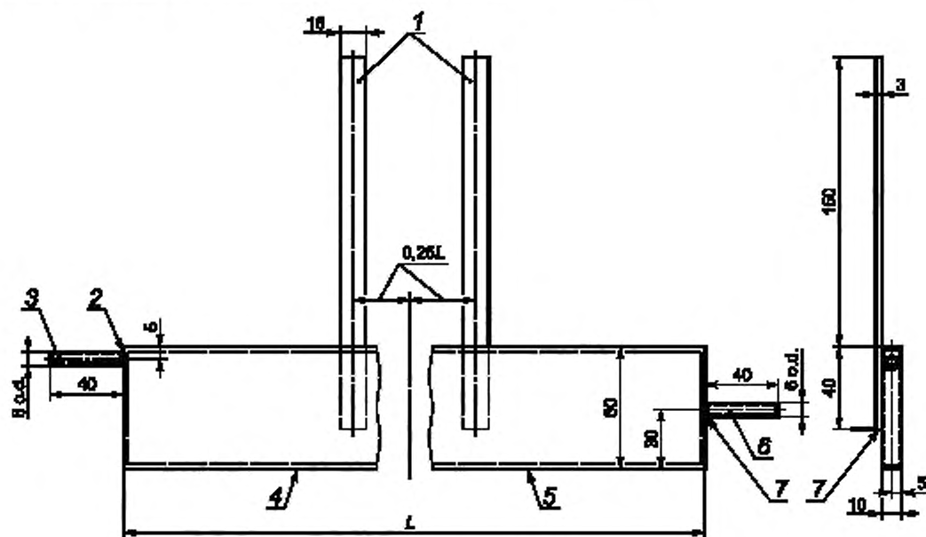
1 — латунь никелированная; 2 — место спайки твердым припоем; 3 — отвод воды, 4 — толщина 1 мм, латунь, с родиевым покрытием; 5 — полированная до блеска поверхность без шероховатостей; 6 — подвод воды, 7 — место спайки твердым припоем
