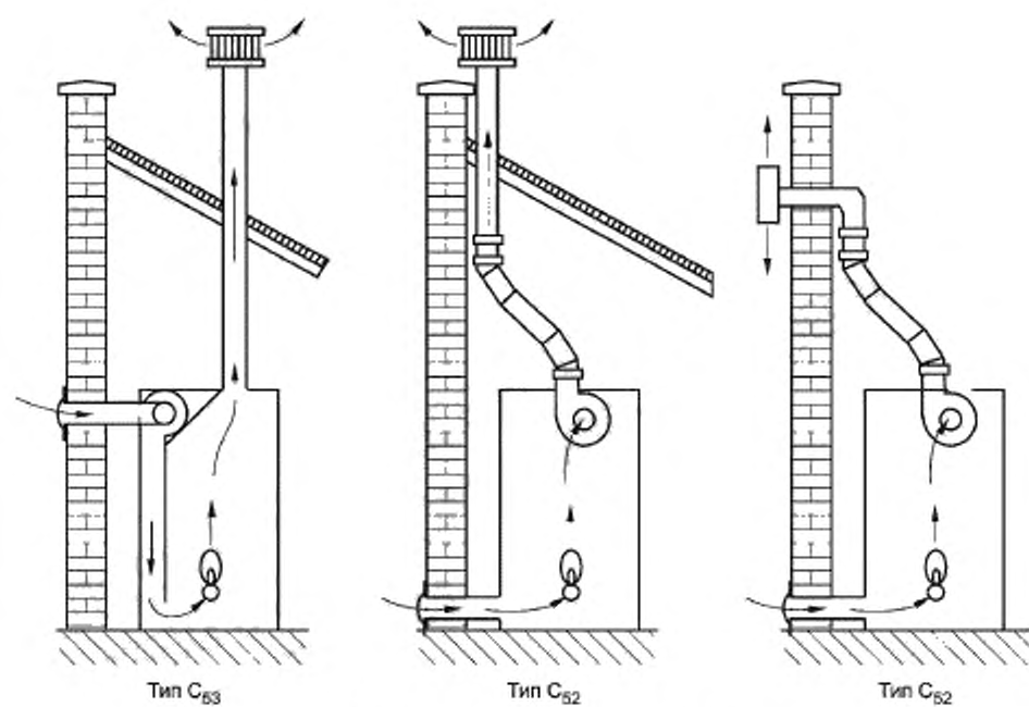
Рисунок В.5 — Схемы приборов типа C 5
