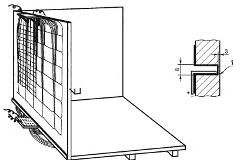
а) расположение термопар
