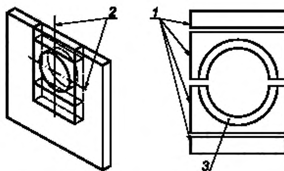
а) расположение термопар
