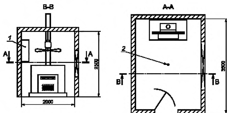
1 — кондиционер; 2 — место отбора проб в геометрическом центре испытательной камеры
