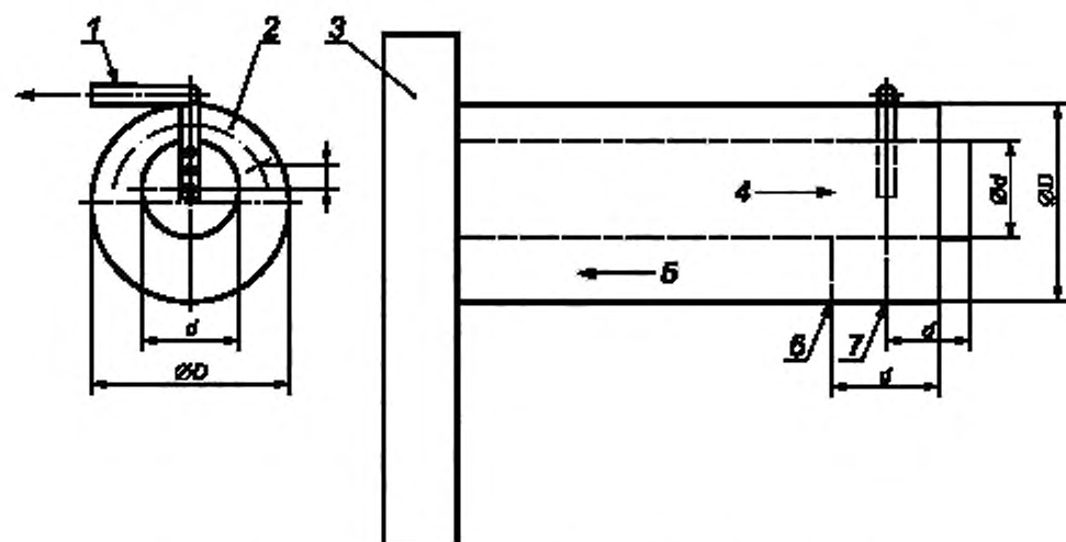
1 — преобогреватель; 2 — воздух для горения; 3 — камера сгорания; 4 — продукты сгорания; 5 — воздух; 6 — сечение для измерения температуры воздуха для горения; 7 — сечение для измерения температуры продуктов сгорания и дымохода
