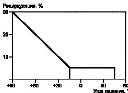
Рисунок С.1 — Максимальная допустимая рециркуляция продуктов сгорания
