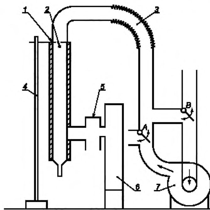
1 - испытательный дымоход (см. рисунок 1); 2 - место измерения тяги; 3 - гибкий трубопровод; 4 - опорная стойка; 5 - испытуемый прибор; 6 - вентилятор; 7 - воздуходувка; А, В - заслонки клапанов для получения нормальной и обратной тяги
