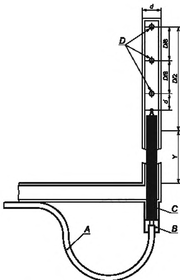
А — провод хромо-алюминиевой термопары; В — изолирующий материал; С — керамическая втулка с двойным отверстием; D — три отверстия для отбора проб \varnothing X мм
