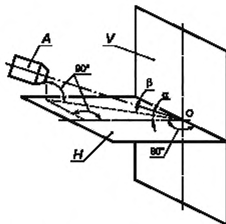
A — вентилятор; H — горизонтальная плоскость, V — вертикальная плоскость; \alpha = 0^\circ (горизонтальный воздушный поток), плюс 30^\circ и минус 30^\circ ; \beta = 0^\circ (отраженный воздушный поток), 15^\circ, 30^\circ, 45^\circ, 60^\circ, 75^\circ, 90^\circ (перпендикулярно испытательной стенке)
