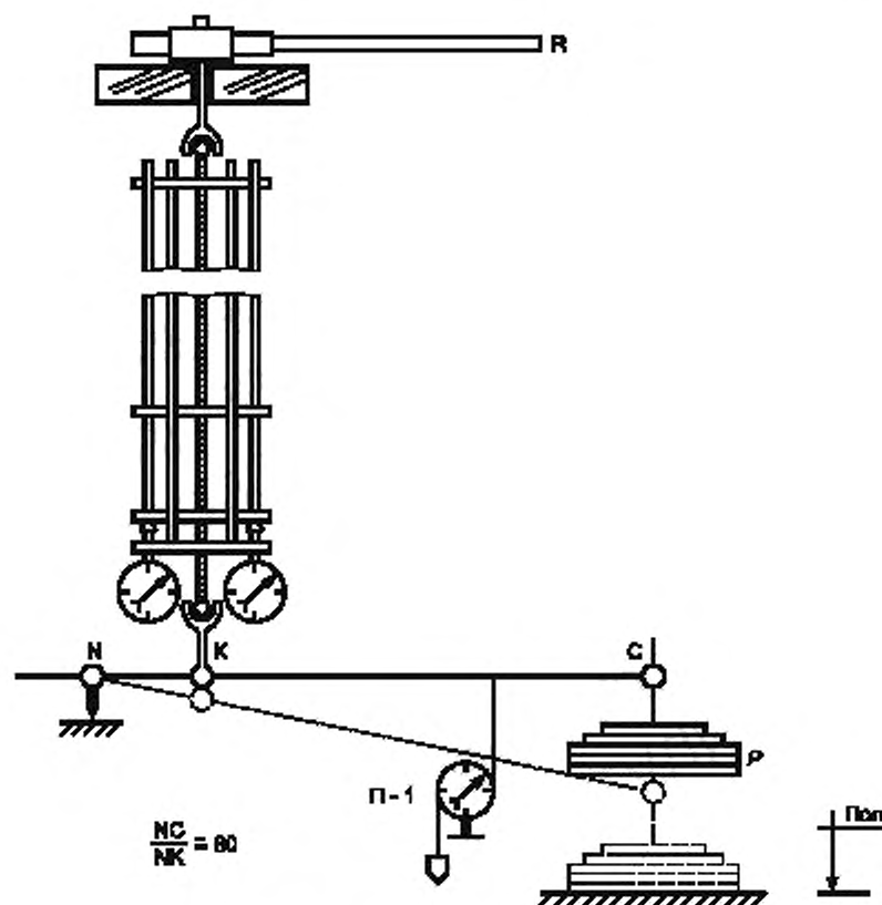
Рисунок 6.2 — Схема испытания образцов
