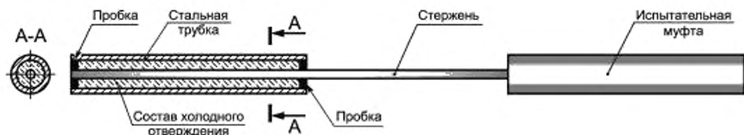
Рисунок 5.1 — Вид типового образца для испытаний
