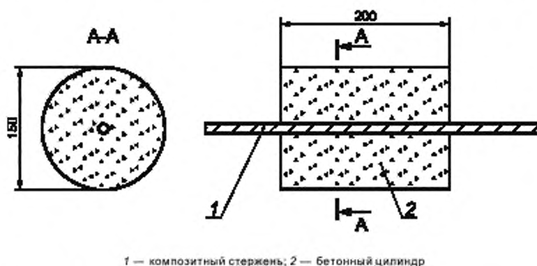
Рисунок 6.1 — Типовые размеры бетонного цилиндра с установленным стержнем
