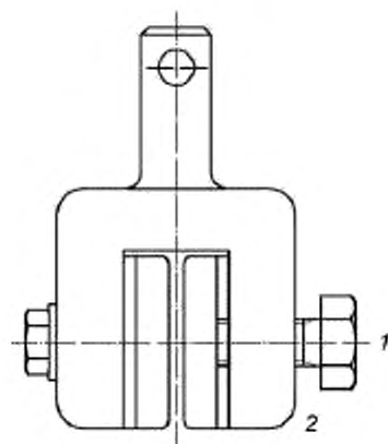
1 – сжимающее усилие, регулируемое до 400 кН; 2 – максимальная ширина образца для испытания: 0,5 м
