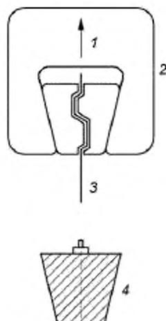
1 – направление прилагаемого усилия; 2 – зубчатый клин; 3 – геосинтетический материал; 4 – клин из эпоксидной смолы или мягкого металла
