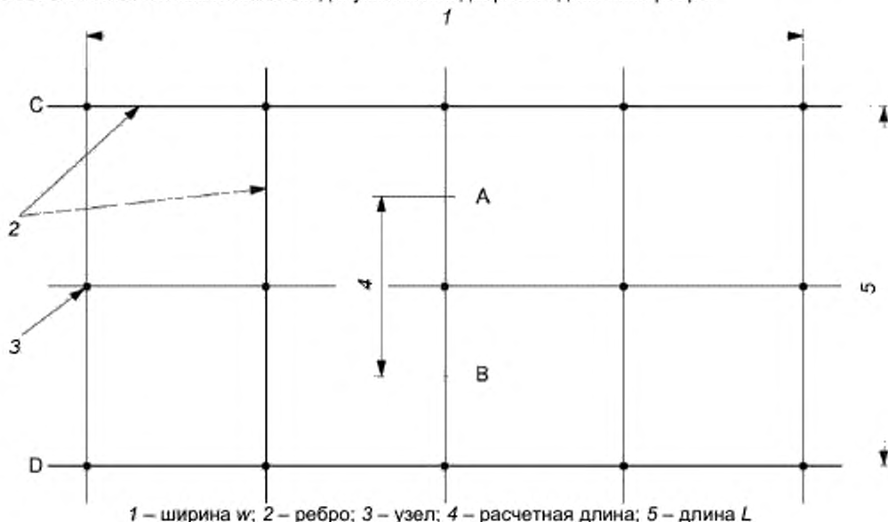
Рисунок 7 – Стандартная георешетка
