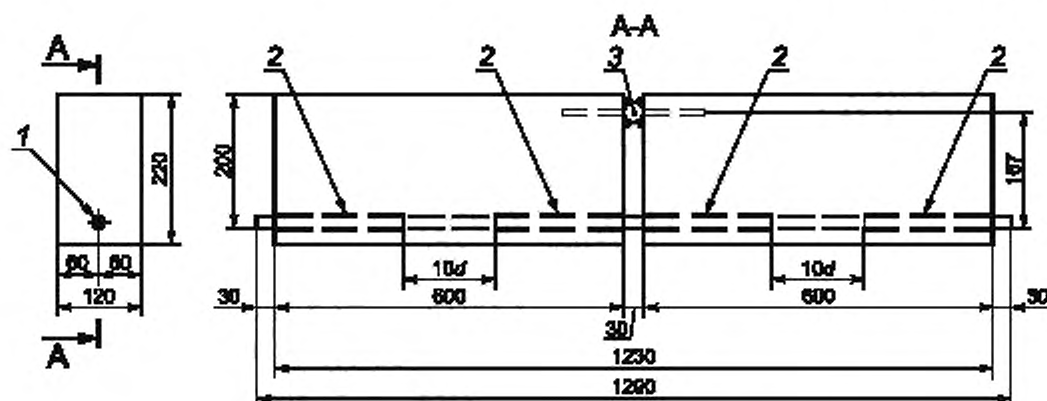
1 — стержень; 2 — поливинилхлоридная трубка; 3 — стальной цилиндр
