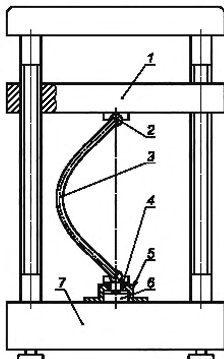
1 — подвижная traverse испытательной машины; 2 — верхняя шарнирная опора; 3 — образец-стержень; 4 — нижняя шарнирная опора; 5 — корпус силоизмерительного узла; 6 — датчик силы; 7 — станина испытательной машины
