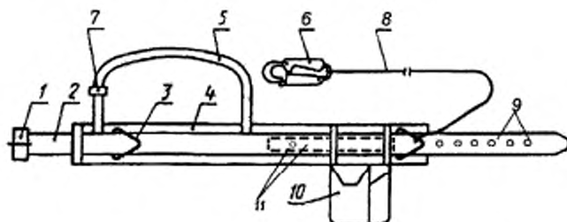
1 — пряжка со шпеньком; 2 — ремень; 3 — боковое кольцо; 4 — кушак; 5 — наплечная лямка; 6 — карабин; 7 — пряжка лямки; 8 — фал; 9 — люверсы; 10 — сумка для инструмента; 11 — амортизатор с чехлом и контрольным люверсом
