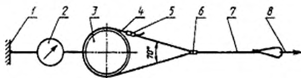
1 — жесткая опора; 2 — измеритель усилия; 3 — цилиндр диаметром 300 мм; 4 — пояс; 5 — пряжка пояса; 6 — боковое кольцо пояса; 7 — строп; 8 — растягивающее усилие
