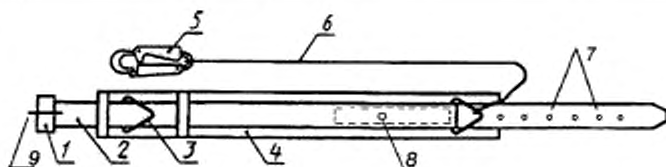
1 — пряжка; 2 — ремень; 3 — боковое кольцо; 4 — кушак; 5 — карабин; 6 — фал; 7 — люверсы, 8 — амортизатор с чехлом и контрольным люверсом, 9 — шпенец
