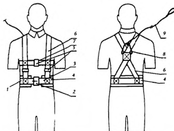
1 — ремень; 2 — пряжка со шпеньком; 3 — люверсы; 4 — кушак; 5 — пряжка наплечной и нагрудной лямок; 6 — наплечная лямка; 7 — нагрудная лямка; 8 — распределительное кольцо; 9 — веревка
