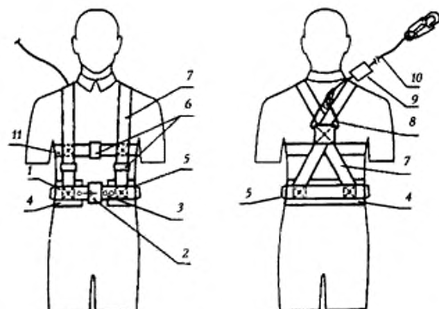
1 — ремень; 2 — пряжка со шпеньком; 3 — люверсы; 4 — кушак; 5 — боковое кольцо; 6 — пряжка ремня и лямки; 7 — наплечная лямка; 8 — распределительное кольцо; 9 — амортизатор; 10 — фал с карабином (строп); 11 — дублирующий ремень
