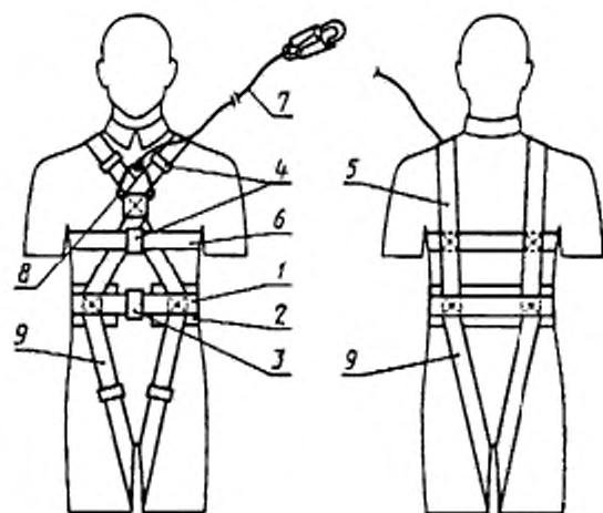
Рисунок 5 — Лямочный пояс, тип Д (Да)
