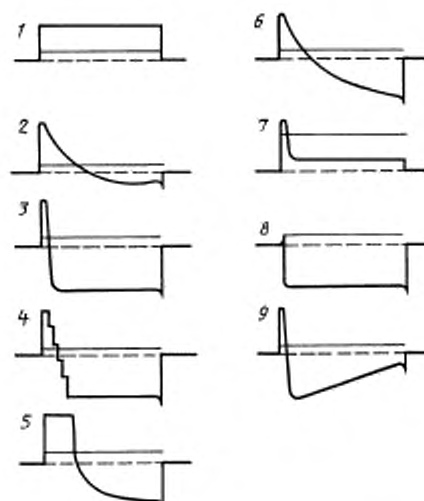
1 — несмачивание; 2 — плохое смачивание; 3 — хорошее смачивание; 4 — быстрое смачивание, ограниченное тепловыми требованиями; 5 — замедленное смачивание; 6 — медленное смачивание; 7 — выталкиваемый образец; 8 — очень быстрое смачивание; 9 — нестабильное смачивание
