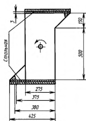
Вращающийся барабан (со стальной плитой толщиной 3 мм)
