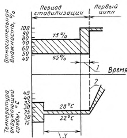
Испытание Db. Период стабилизации
