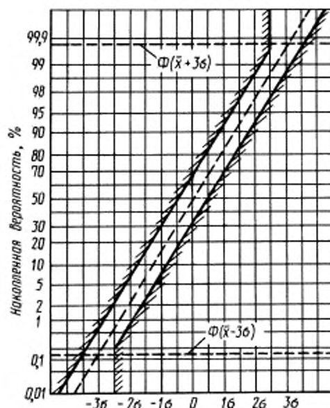
Зона допусков для распределения мгновенных значений ускорения
