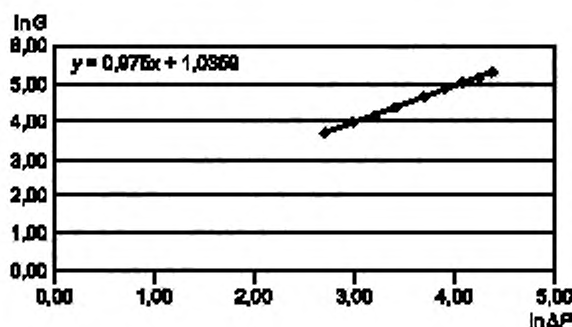
Рисунок А.1 — Графическое определение параметров уравнения воздухопроницаемости образца каменной ваты
