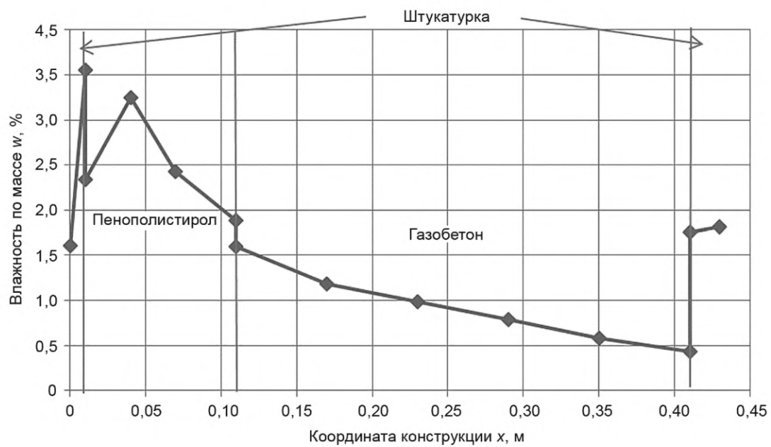
Рисунок А.1 — Распределение влажности внутри конструкции
