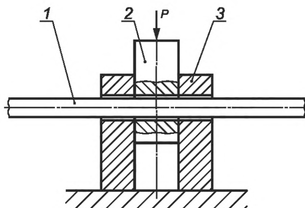
1 — испытательный образец; 2 — верхний нож; 3 — нижние ножи
