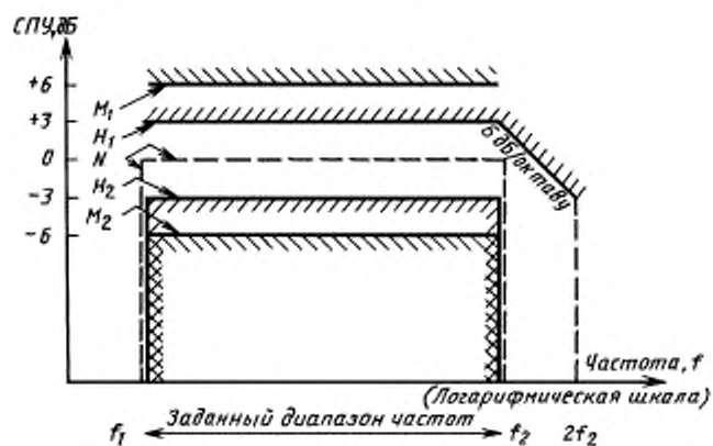
Спектр плотности ускорения (СПУ) и границы допусков
