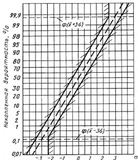
Зона допусков для распределения мгновенных значений ускорения
