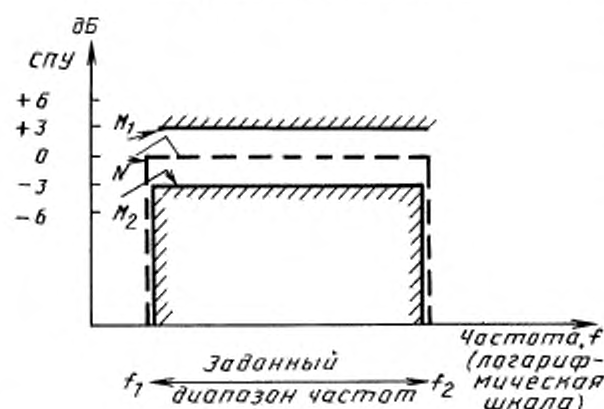
Спектр СПУ и диапазон допусков
