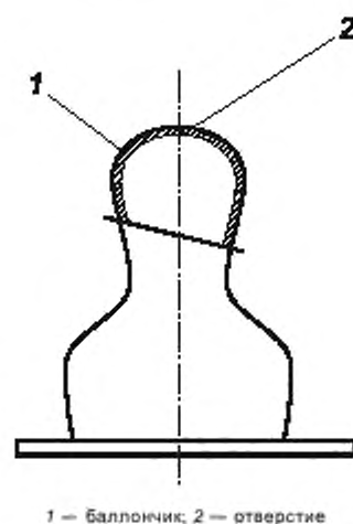
Рисунок 1 — Конструкция соски
