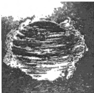
Рисунок 4 — Типичные пятна износа шарика перед удалением налипшего металла
