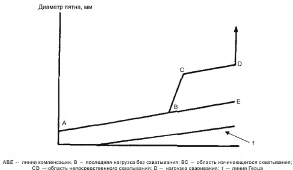
Рисунок 1 — График зависимости значения диаметра пятна износа от прилагаемой нагрузки
