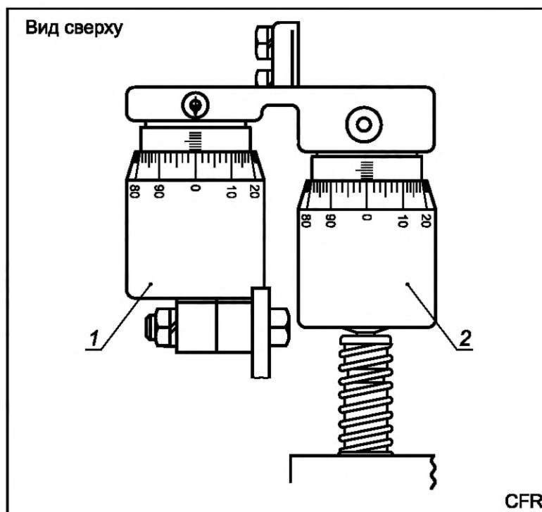
1 — регулировка момента впрыска; 2 — расход топлива
