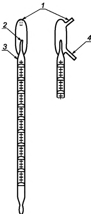
1 — вентиляционная трубка; 2 — автоматический нуль; 3 — градуировка, начинающаяся с 3 %; 4 — трубка для слива избытка топлива
