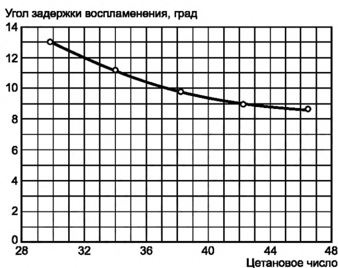
Рисунок Г.4.1 — Зависимость угла задержки воспламенения от цетанового числа
