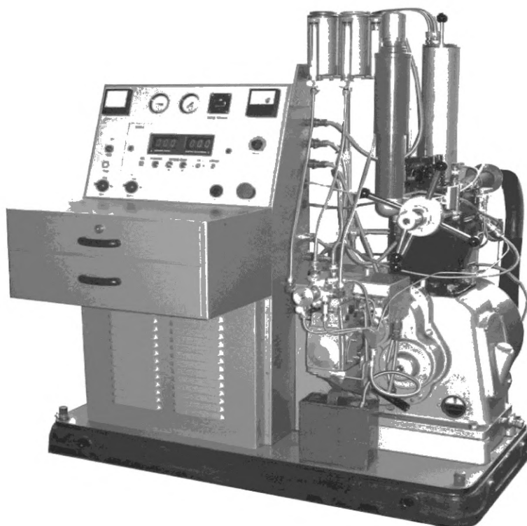
Рисунок 2 — Установка ИДТ-90 для определения цетанового числа
