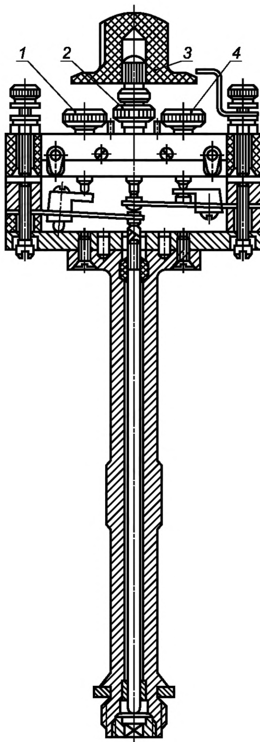
Рисунок Д.2.2 — Продольный разрез индикатора воспламенения
