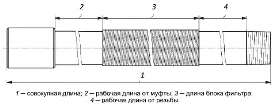
Рисунок D.2 — Комплект с одним противопесочным фильтром
