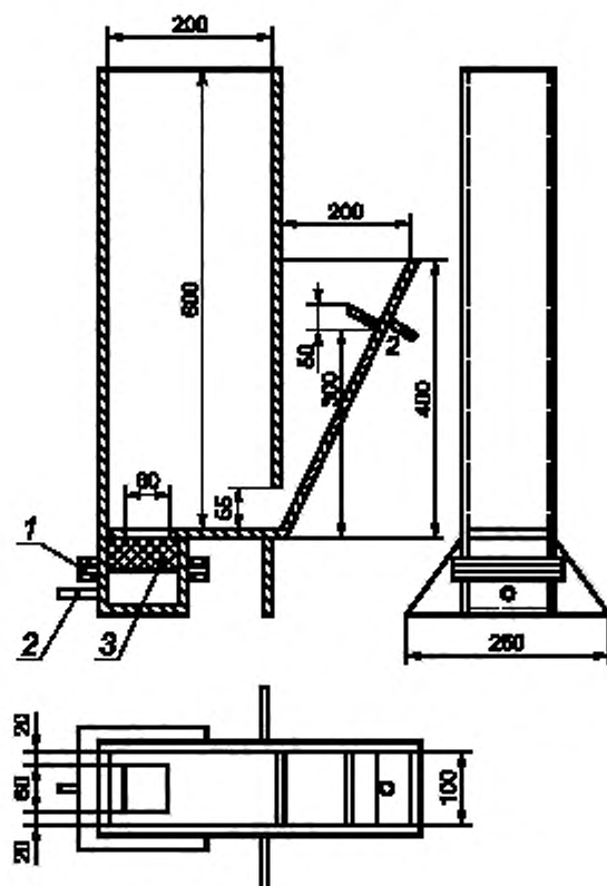
Схема модельного аэротенка-отстойника
