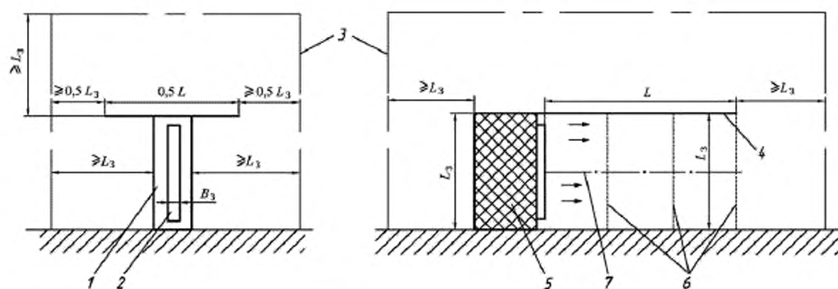
1 — завеса; 2 — сопло завесы; 3 — стены помещения; 4 — верхняя ограждающая стенка; 5 — всасывающее окно завесы; 6 — сечения в вертикальной плоскости для измерения эпюры скорости; 7 — сечение в горизонтальной плоскости для измерения эпюры скорости
