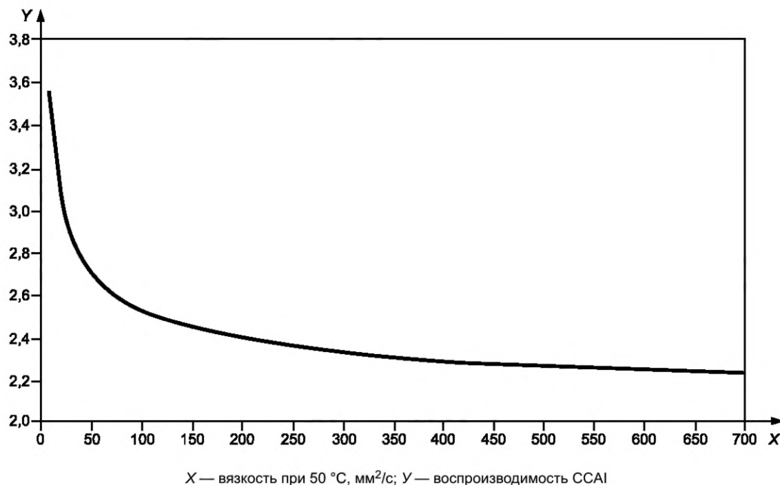
Рисунок Б.2 — График воспроизводимости определения CCAI в зависимости от значения вязкости
