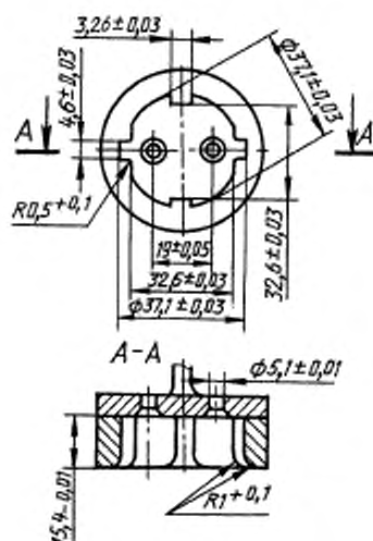
Рисунок Б.21 — Калибр для проверки размеров вилок с боковым заземляющим контактом
