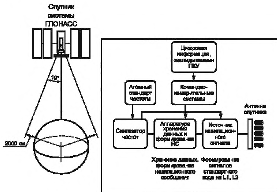
Рисунок А.1 — Процесс генерации сигналов на спутнике
