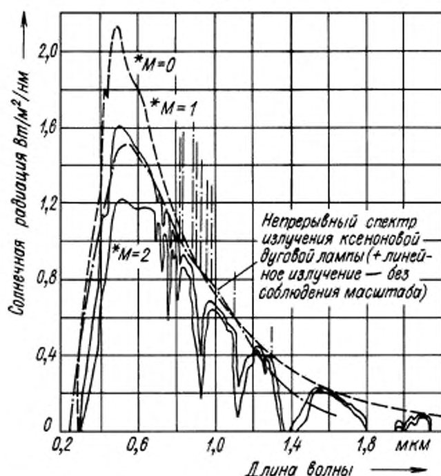
Сравнение излучения типичной ксеноновой дуговой лампы высокого давления с кривыми спектрального распределения солнечного излучения для воздушных масс 0—1 и 2
