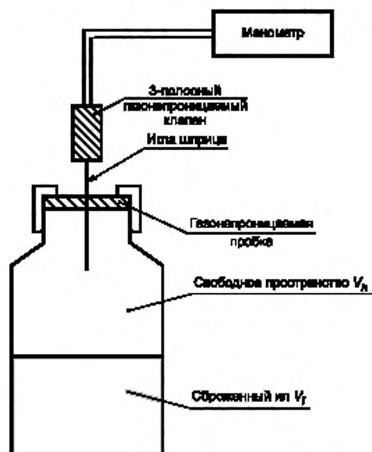
Рисунок А.1 — Тестовые сосуды при температуре (35 \pm 2) ^\circ\text{C}
