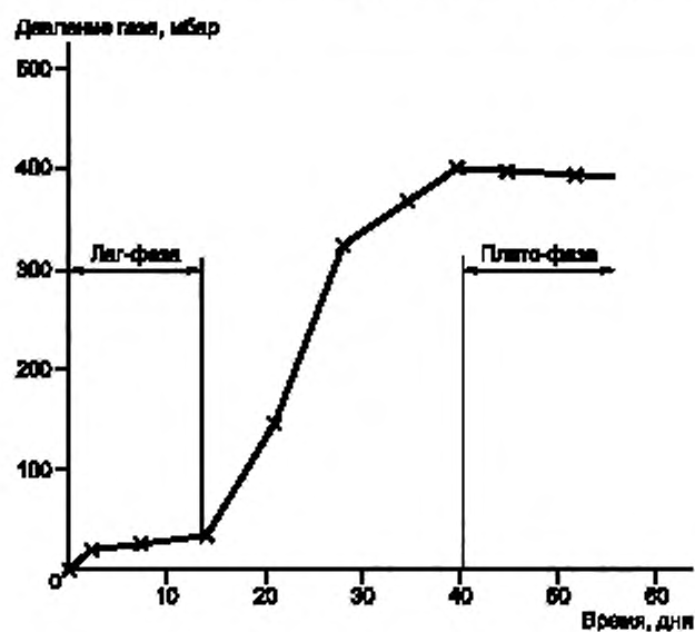
Рисунок В.1 — Пример кривой биоразложения
