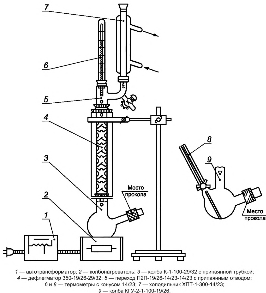
Рисунок 2 — Установка для определения массовой доли пропеллента
