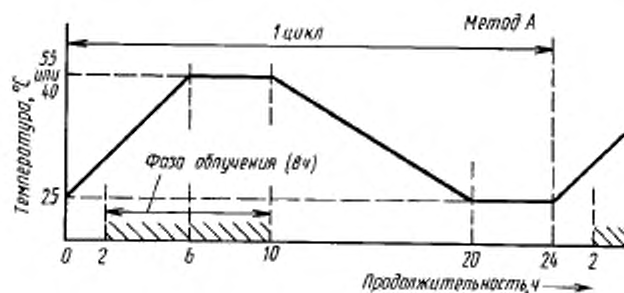
Режим облучения и зависимость температуры от времени
