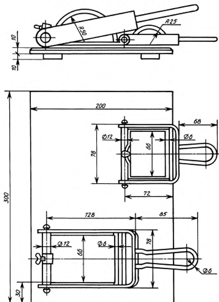
Прибор для определения эластичности шпатлевок при изгибе
