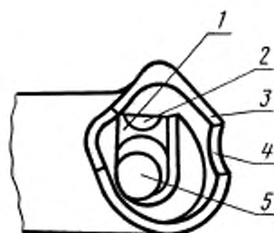
1 — головка (вращающаяся); 2 — прорезь для вставления провода; 3 — втулка; 4 — выемка для удержания провода; 5 — отверстие для размещения вывода
