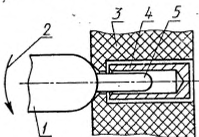
1 — рукоятка; 2 — изгибающий момент; 3 — изолятор соединителя; 4 — гнездовой контакт; 5 — испытательный штырь
