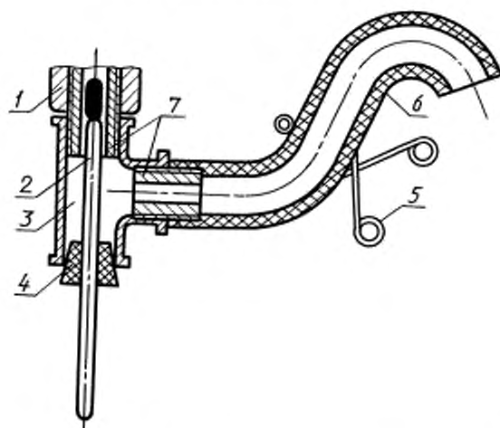
Прибор для измерения температуры
