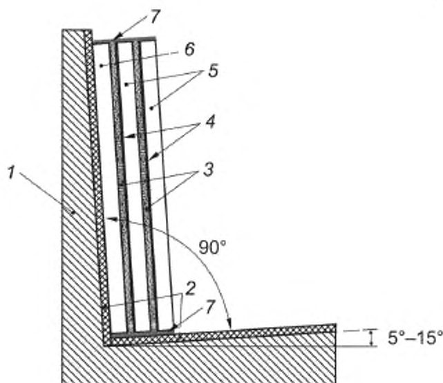
1 – опора; 2 – резиновые или войлочные подкладки; 3 – прокладочный материал; 4 – покрытие на стекле; 5 – стекло с мягким покрытием; 6 – лист бесцветного флоат-стекла; 7 – паронепроницаемая клейкая лента с осушителем
