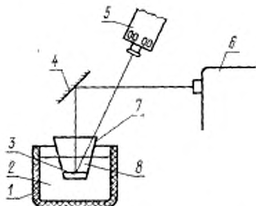
1—плавильная чашка; 2—жидкий азот; 3—анализируемый раствор; 4—зеркало; 5—осветитель; 6—монокроматор; 7—платиновый тигель; 8—жидкий азот.
