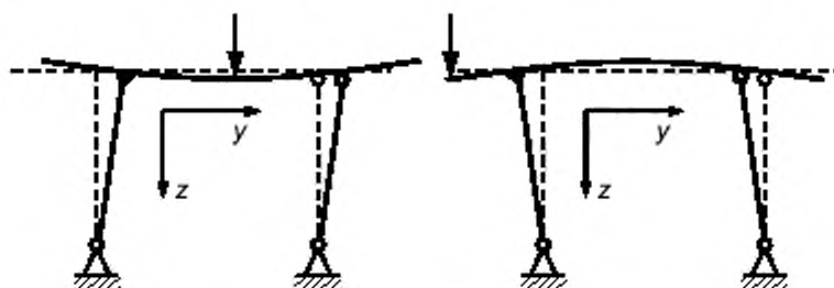
Рисунок 2 – Схемы деформаций металлической конструкции козлового крана
