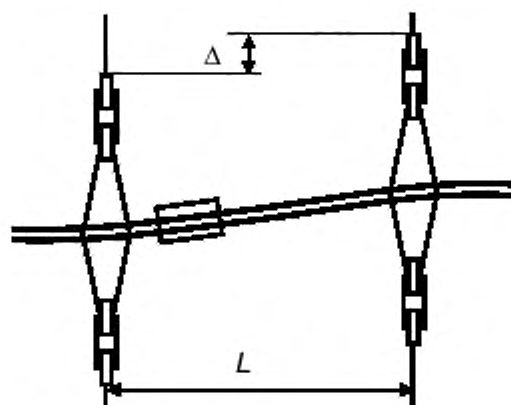
Рисунок 1 – Схемы к определению перекаса
