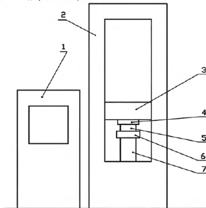
1 — пульт управления машиной; 2 — разрывная машина; 3 — подвижная траверса; 4 — сжимающая плита; 5 — образец; 6 — опорная плита; 7 — силоизмерительный датчик.
