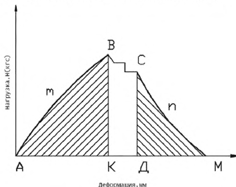
Рисунок Д.2 – Зависимость деформации образца от нагрузки
