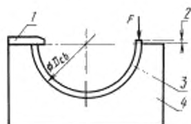
1 — фиксирующий упор; 2 — выступание; 3 — эталонный или испытываемый вкладыш; 4 — контрольный блок
