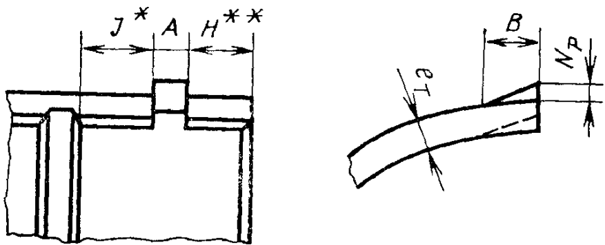
Установочный выступ
