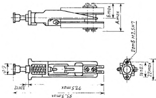
Переключатель ПКТ1
