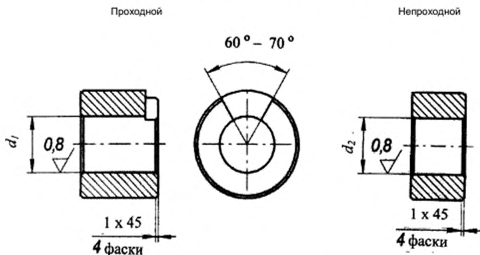
Рисунок А.1 – Проходные и непроходные калибры-кольца для контроля охватываемых концов фитингов
