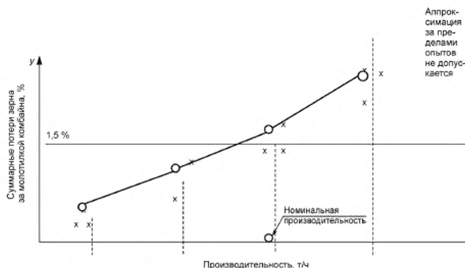
Рисунок 1 — График зависимости суммарных потерь зерна комбайном от производительности
