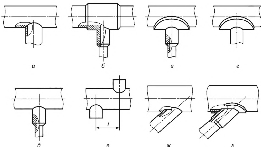
a — без укрепления; б — с помощью тройника; в — укрепленное штуцером и накладкой; г — укрепленное накладкой; д — укрепленное штуцером; е — крестообразное; ж — наклонная врезка без укрепления; з — наклонная врезка с укреплением штуцером и накладкой
