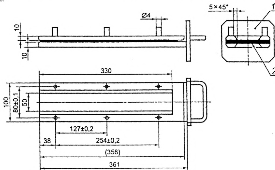
Рисунок 7.20 — Схема подставки
