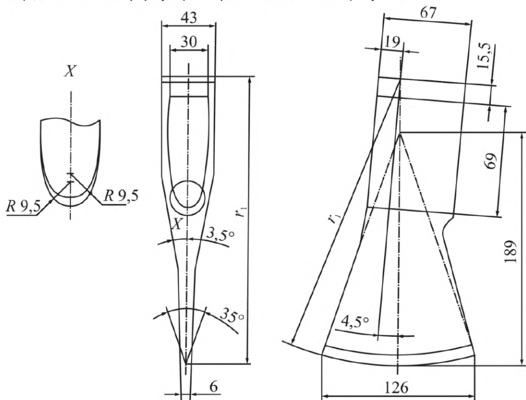
Рисунок 2 – Топор
