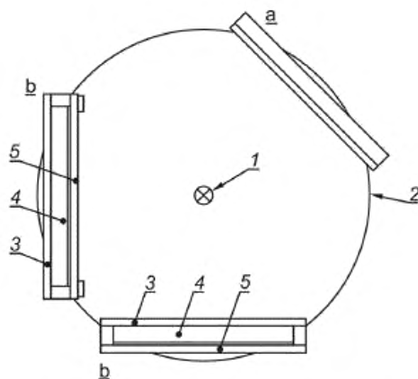
1 – ксеноновая лампа; 2 – круговой держатель; 3 – бесцветное флоат-стекло номинальной толщиной 4 мм; 4 – межстекольное пространство 12 мм; 5 – стекло с покрытием, обращенным внутрь межстекольного пространства; а – контрольный образец стекла; б – образцы для испытаний
