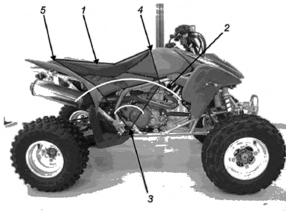
1 — расстояние от площадки для ноги; 2 — траектория движения колена; 3 — площадка для ноги; 4 — крайняя передняя точка, в которую может передвинуться испытательный шаблон; 5 — крайняя задняя точка, в которую может передвинуться испытательный шаблон
