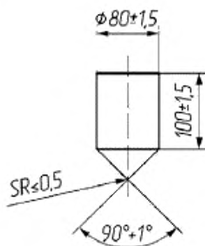
Рисунок G.3 — Испытательный конус
