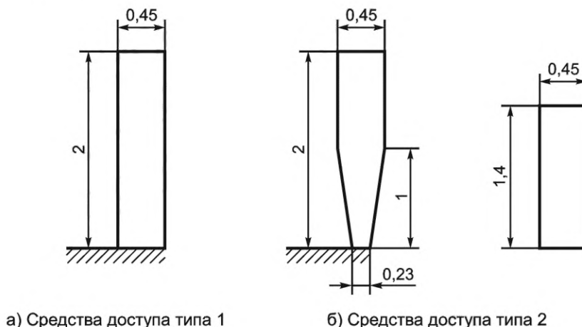
Рисунок 15 — Минимальное свободное пространство (размеры в свету) для проходов и пандусов (размеры в м)
