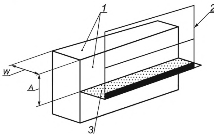
1 — непрерывная поверхность; 2 — перила; 3 — проход; A — высота непрерывной поверхности; W — ширина непрерывной поверхности (к непрерывным поверхностям относятся, в том числе, поверхности, образованные перфорированным листом, сеткой и т. п.)
