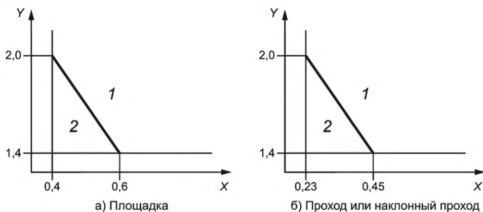
Рисунок 12 — Связь между высотой в свету и шириной площадки или прохода
