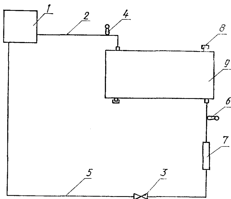
Стенд теплогидравлический
