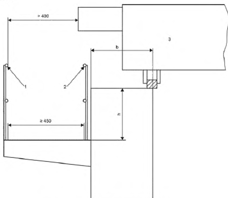
1 – перила А; 2 – перила Б; 3 – тележка
