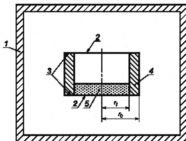
1 — шкаф; 2 — алюминиевая фольга; 3 — клей; 4 — образец; 5 — влагопоглотитель; r_i — внутренний радиус образца; r_o — наружный радиус образца
